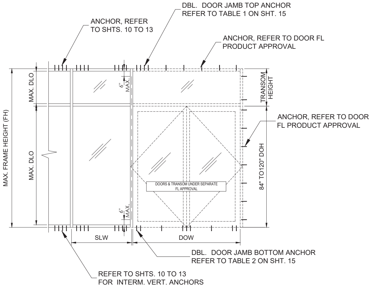
ELEVATION 4
